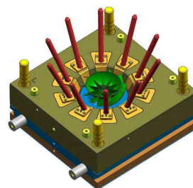
叶轮模具 Impeller mould
